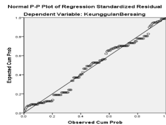
Gambar 3. Uji Normalitas P-Plot.
