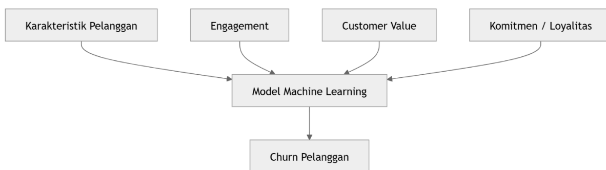
Gambar 1. Kerangka Konseptual.
