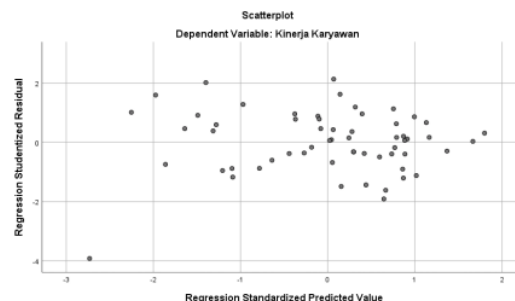
Gambar 2 Uji Heterokedastisitas
