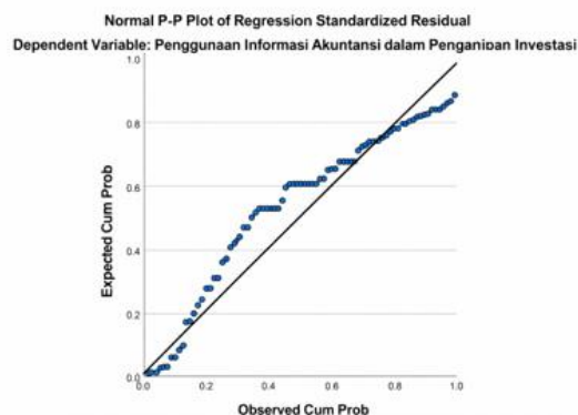
Gambar 1. Gambar Uji Normalitas.
