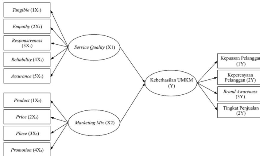
Gambar 1 Kerangka Berpikir
