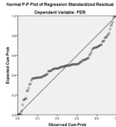
Gambar 2. Normalitas P-Plot
