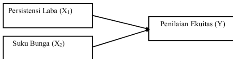
Gambar 1. Kerangka Teoritis
