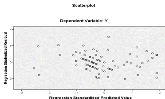
Gambar 2. Diagram Scatterplot Hasil Uji Heteroskedastisitas.
