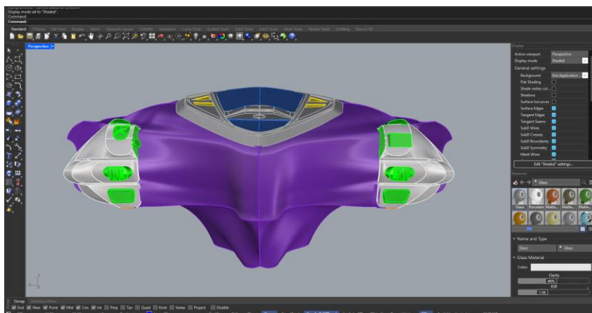
Gambar 8. Digital Prototyping Tombol Kontrol Atas.
